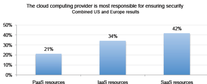
Gambar 5.4 persentase penyediaan layanan cloud computing mengenai keamanan di US dan Eropa
