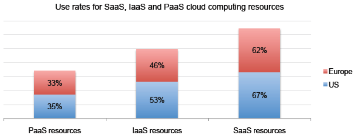
Gambar 5.3 Persentase penggunaan sumber daya cloud computing
