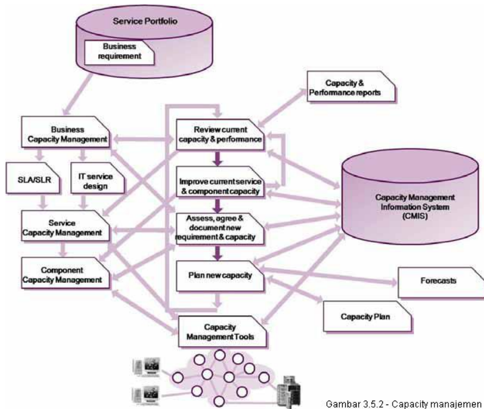
Gambar 3.5.2 - Capacity manajemen
